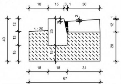
3 Bordstein Granit A2 nach DIN EN 1343 - DIN 482
