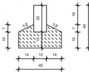
2 Bordstein Granit B6 -120 nach DIN EN 1343 - DIN 482
