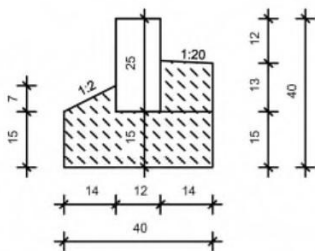
1 Bordstein Granit B6 -120 nach DIN EN 1343 - DIN 482
